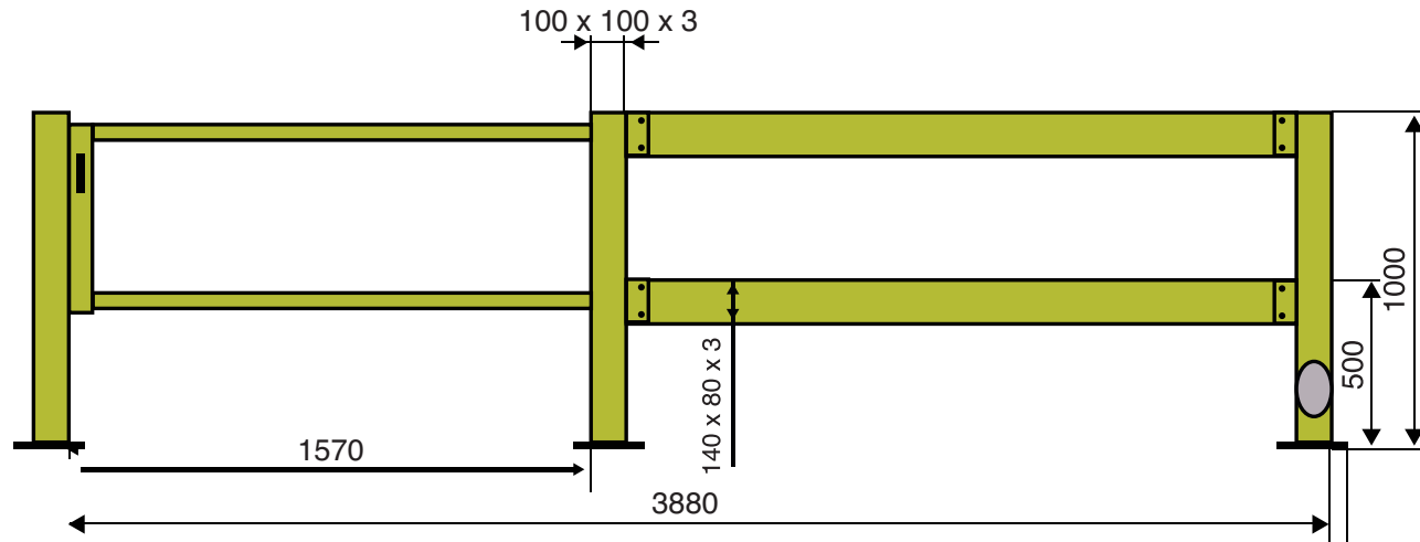
B-B ( 1:18 )
